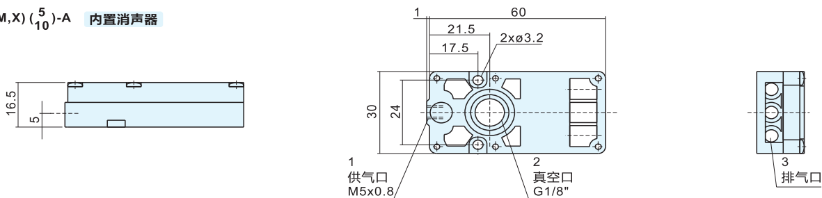
CTL(M,X)( 10 / 20 )-B 内置消声器 5 10 20 30
